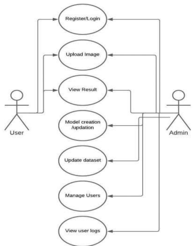
Fig: Use Case Diagram
